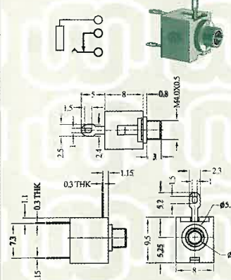
EY-501CM (ø2.5mm Type)
